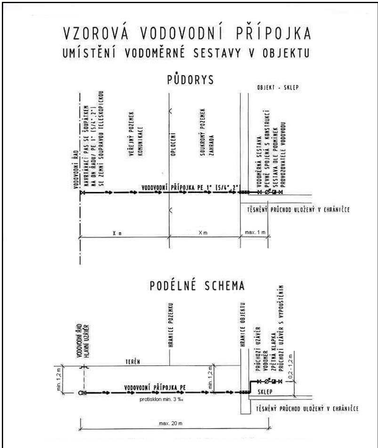
V1 – Vzorová vodovodní přípojka, umístění vodoměrné sestavy v objektu
