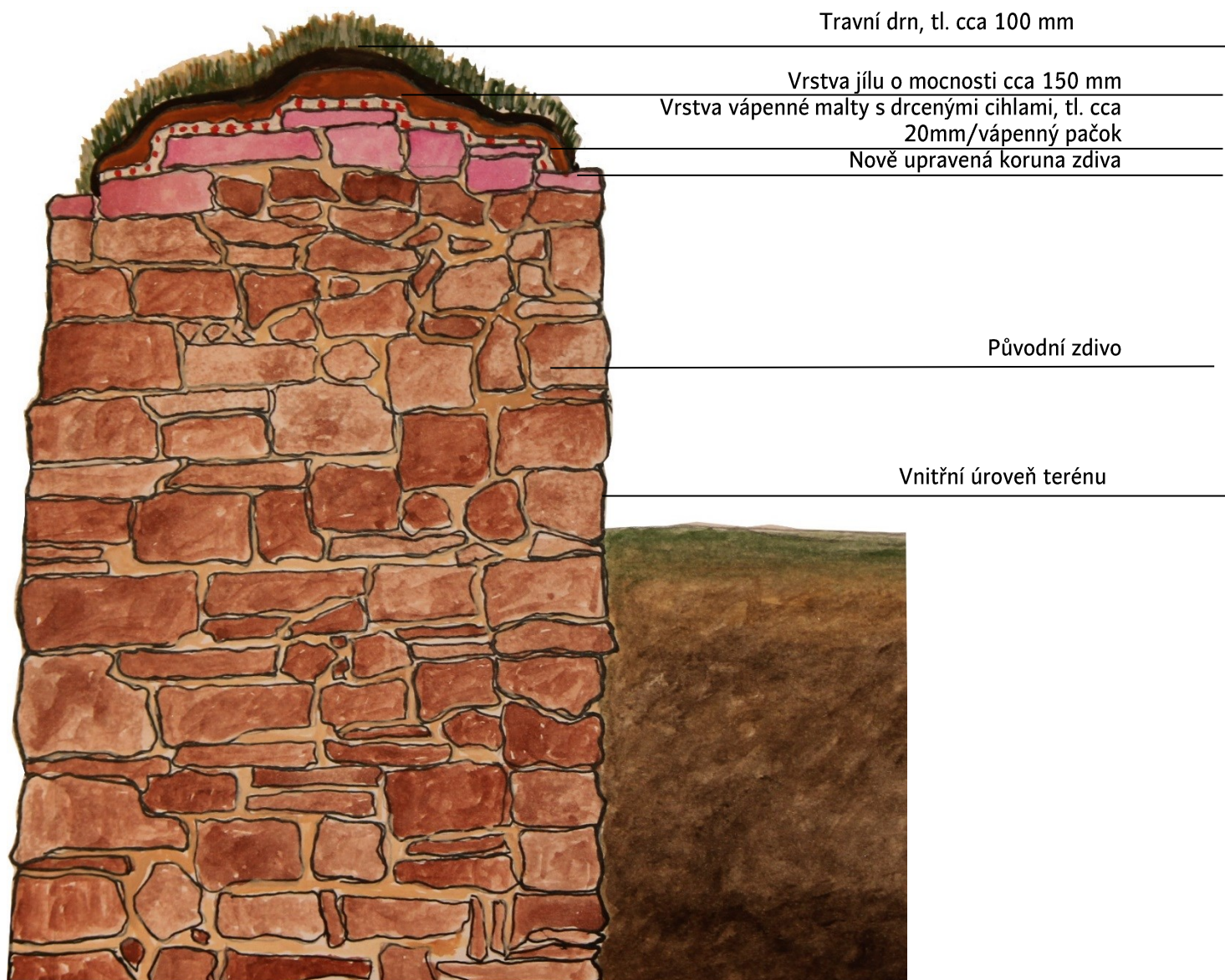
Obr. 2. Řez stěnou hradební zdi: Skladba drnového krytu koruny zdiva městského opevnění v Českém Brodě dle přiloženého návrhu
