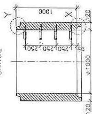
SKRUŽ
