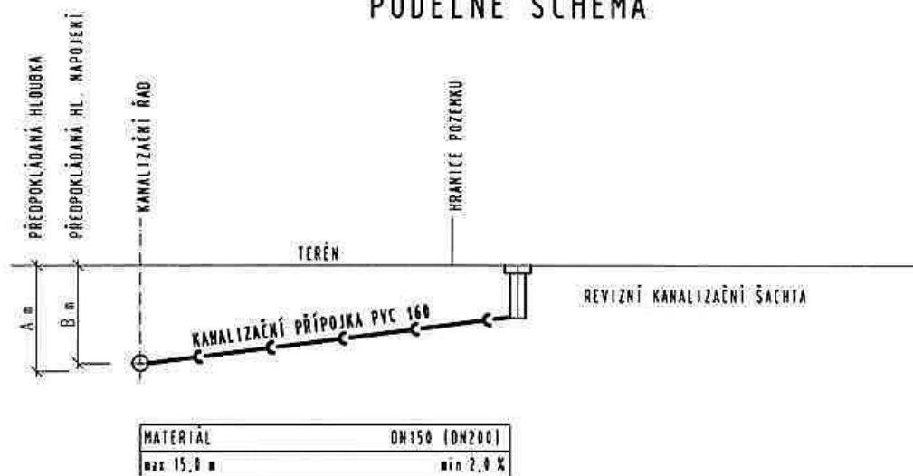
PODÉLNÉ SCHEMA
