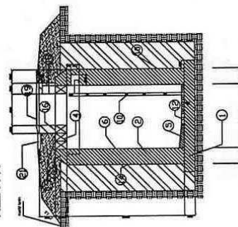
ŘEZ A-A'
