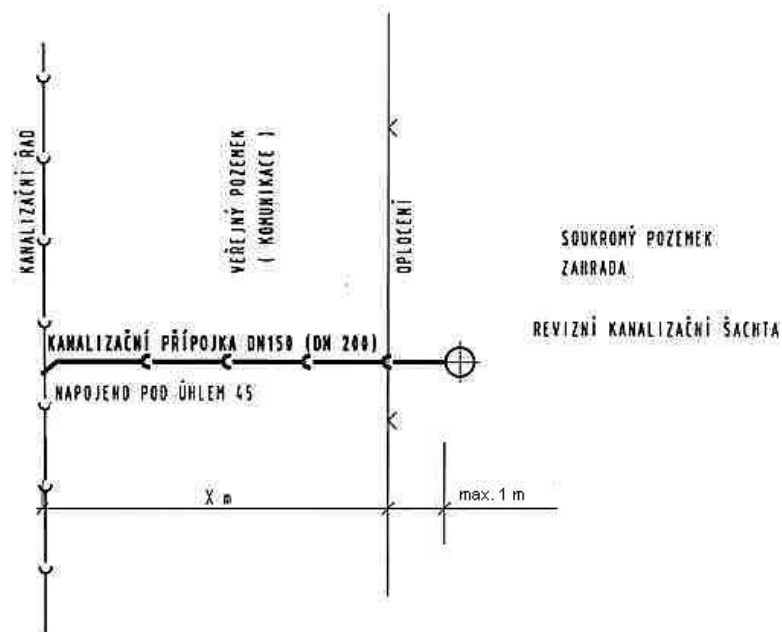
PODÉLNÉ SCHEMA
