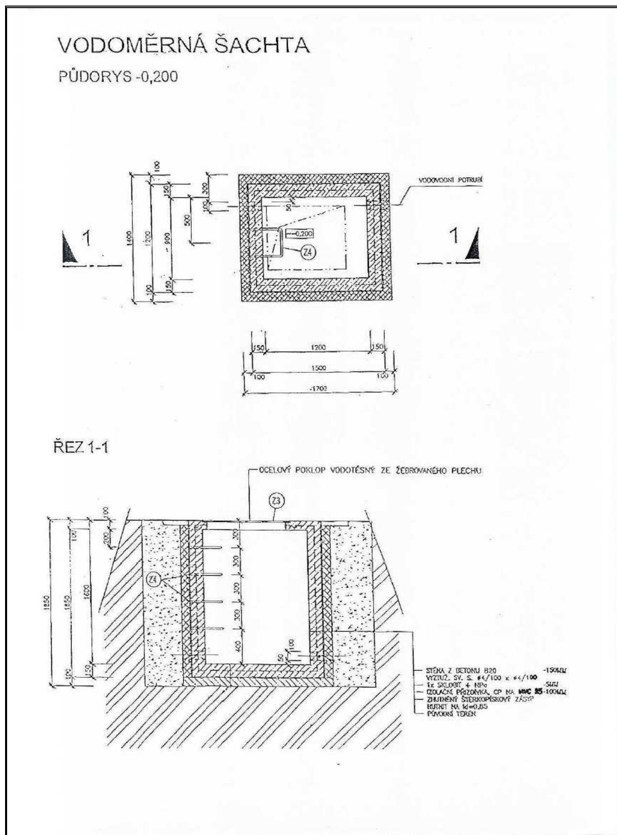
V10 – Vzorový výkres vodoměrné (armaturní) šachty v komunikaci
